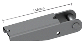
DOBRADIÇA DO TOMBADOR SUPERIOR MOD. NOVO "BRASILIS" 155MM
