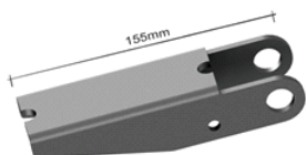
DOBRADIÇA DO TOMBADOR INFERIOR MOD. NOVO "BRASILIS" 155MM
